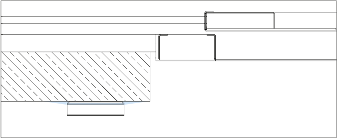
Horizontální řez kabinovými a šachetními dveřmi s dveřní zárubní / Napojení na zeď T1 / ovládací tablo BT-TP-A-100.
